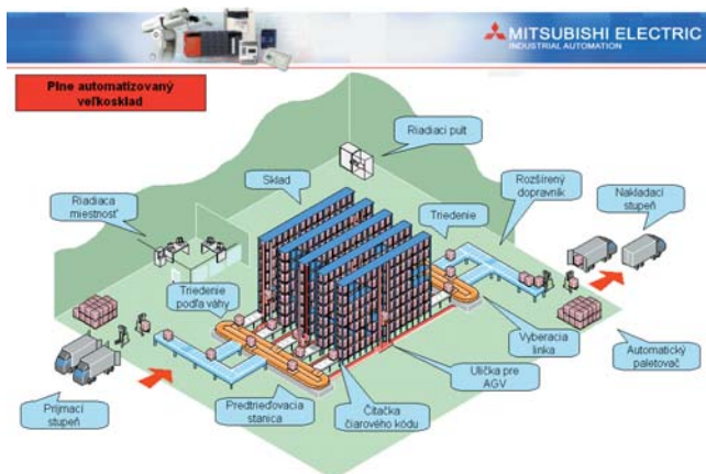
Prehľadová schéma plne automatizovaného veľkoskladu
