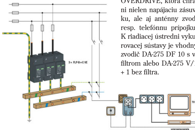
Obr.3 Ochrana elektroniky v RD
