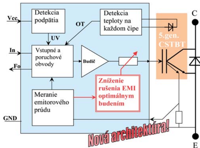
Štruktúra novej generácie IPM modulov série L
