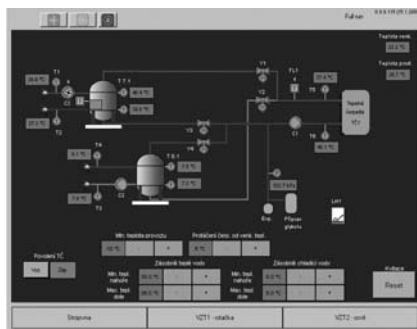
Snímek z displeje dotykového panelu s částí zdrojů
