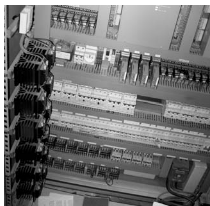
Proudové ventily musely být pro nedostatek místa v rozvaděčích montovány na vnitřní boční stěnu skříně
