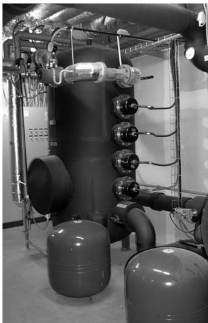
Akumulační nádoba topení 1600 l s elektrickými topnými patronami
