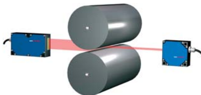
Kontrola nastavenia valcov s ODC
