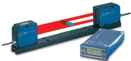
ODC 2500 – 36 mm meria priemer
