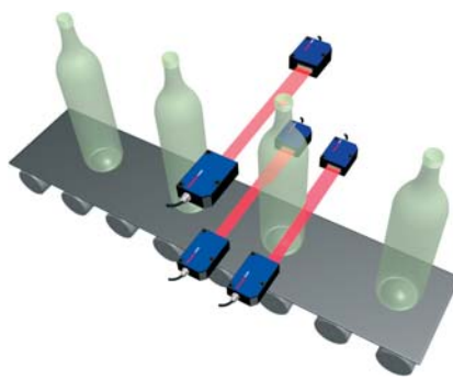
Kontrola rozmerov fliaš s ODC
