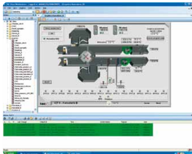
Vizualizácia vzduchotechnických jednotiek v TAC Vista
